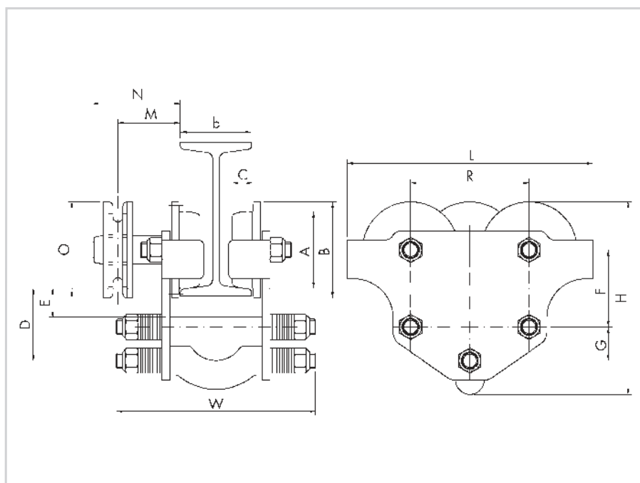
Rollfahrwerk RFW-V
